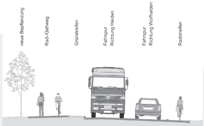
Querschnitt mit Neuaufteilung des Strassenraums
